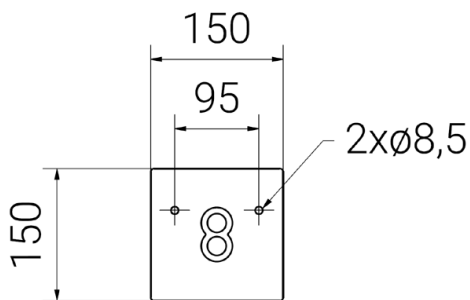
Bild oben: Bodenflansch des 1m Poller
