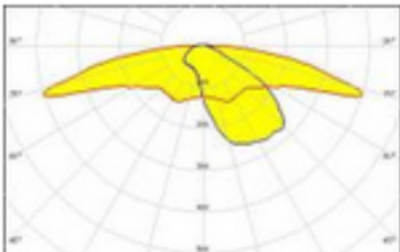
Bild oben: 1m Poller optimiert für Wege
