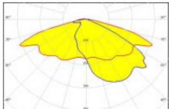
Bild oben: 3m Leuchte Optimiert für Plätze
